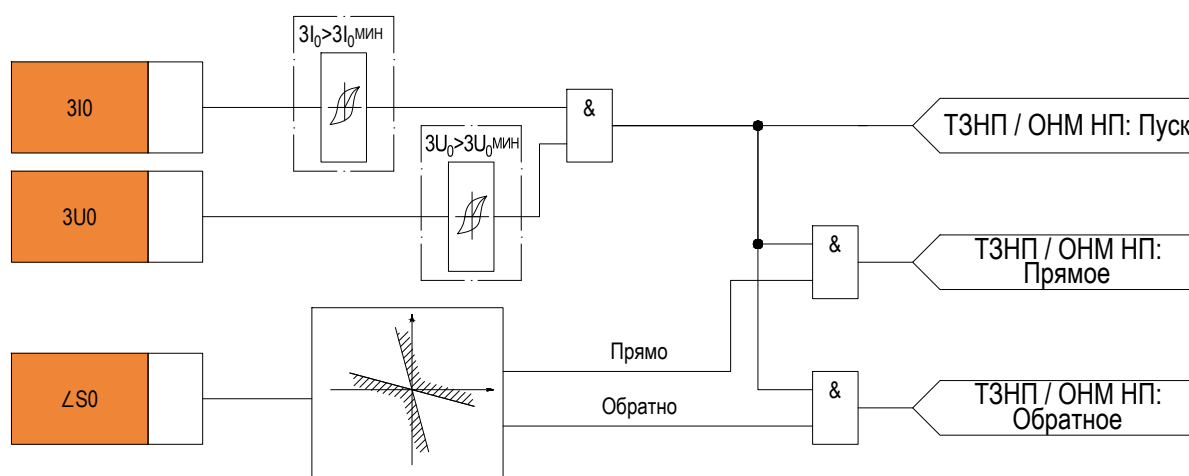
Рисунок 2.32 – Функциональная схема «ОНМ НП»
