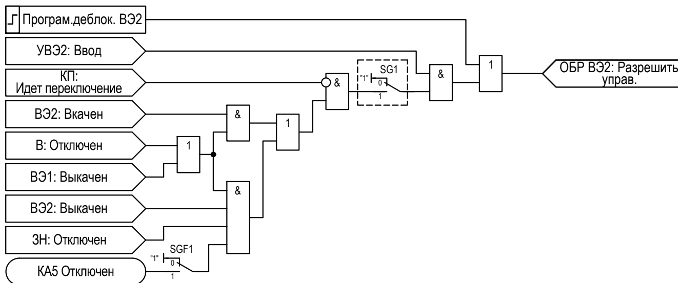
Рисунок 2.68 – Функциональная схема «ОБР ВЭ2»
