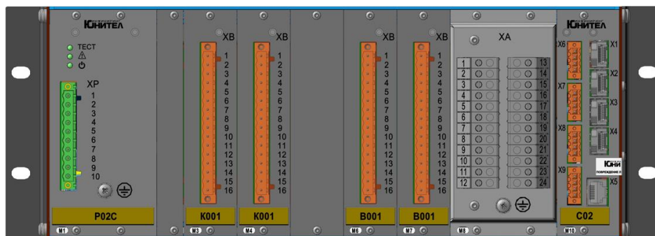
Рисунок 1.1 – Вид устройства «ЮНИТ-М314-ВВ» с размещением модулей по слотам
